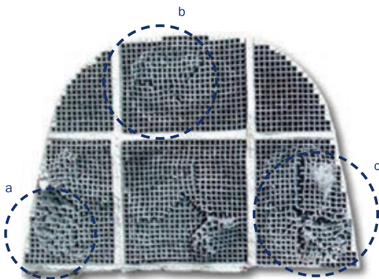
Fig.5 - a,b,c: ZONE DI PARZIALE FUSIONE DEL FILTRO
