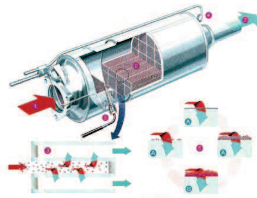
Fig.1 - Il gas entra nei canali aperti ed è costretto ad attraversare le pareti porose dove lascia il particolato uscendo pulito.
