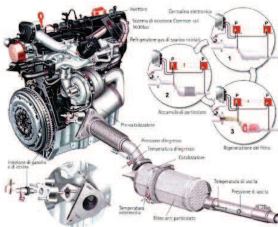
Fig.3 - SISTEMA FAP
